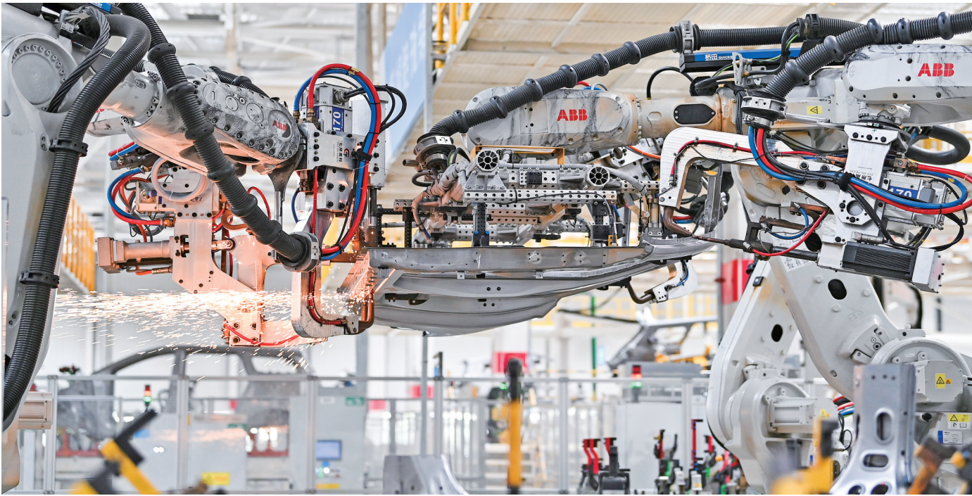
在位于山西省运城经济技术开发区的大运新能源汽车生产基地，智能焊接机器人在作业。
