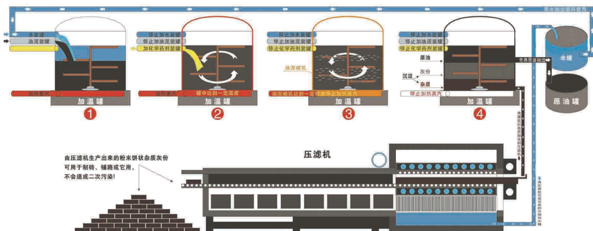
矿物油废弃物环保治理工艺流程图
