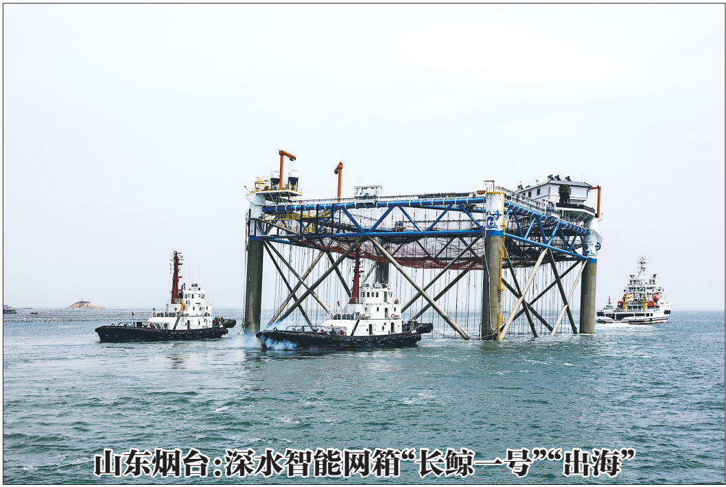
5月8日,“长鲸一号”深水智能网箱被拖带出烟台中集来福士码头,前往烟台长岛海域。“长鲸一号”深水智能网箱长宽均为66米,有效养殖水体为6.4万立方米。网箱配备投饵等自动化设备,可通过大数据技术实时反馈海洋水文信息等。
