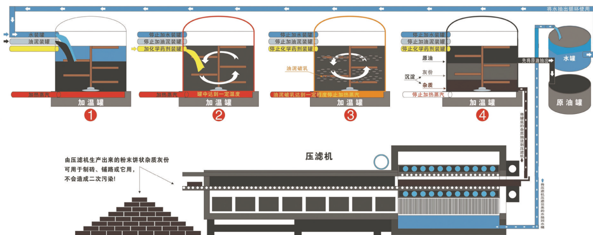
矿物油废弃物环保治理工艺流程图
