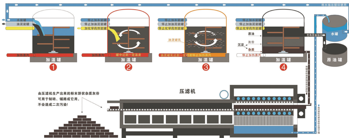
矿物油废弃物环保治理工艺流程图
